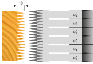
Giunto orizzontale | Horizontal joint
