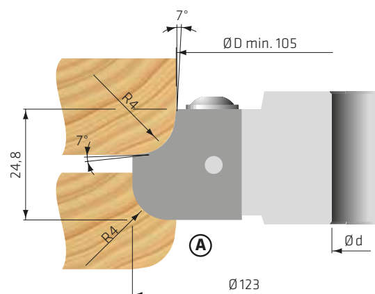
Profilo montato di serie Standard mounted knives
