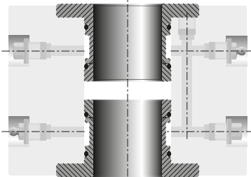
Pressione di serraggio massima: Maximum bush clamping pressure: 400 Bar
