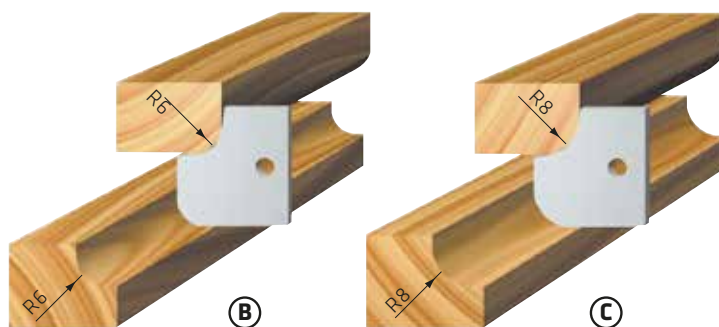
Profili di ricambio Spare knives
