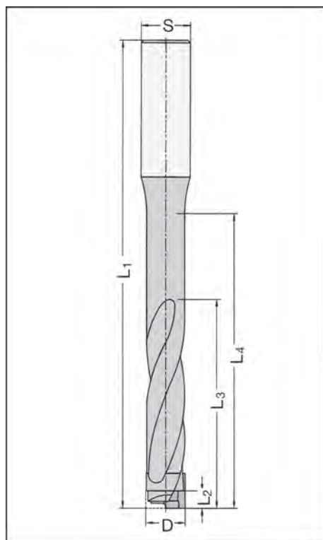
HW-Einbohrmesser
