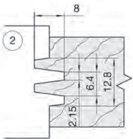
Standardprofile (1:1)
