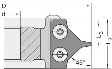
Fasefräser Größe 3
