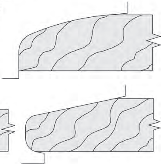
Profilbeispiele (1:1)
